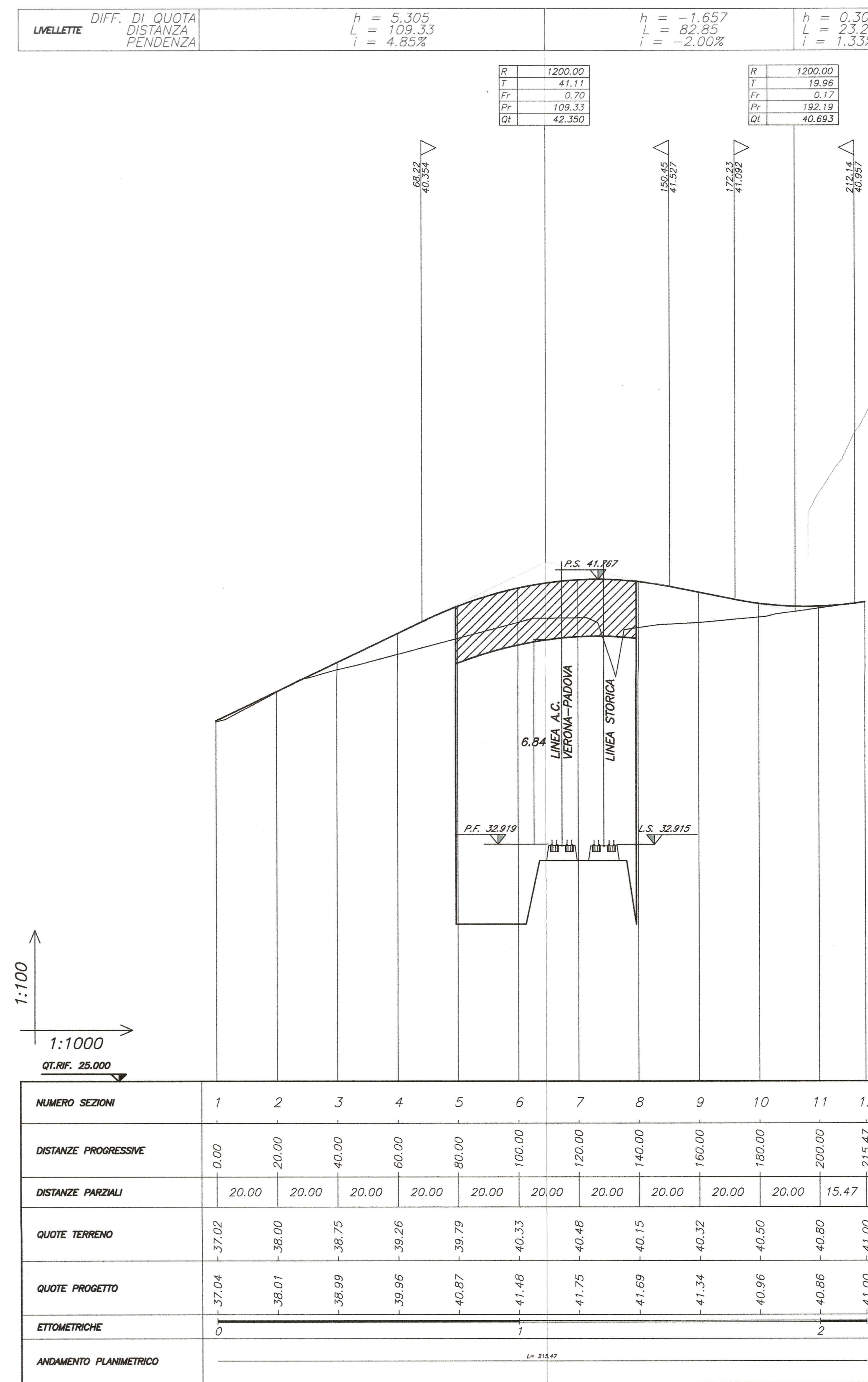
SEZIONE TIPO scala 1:100
