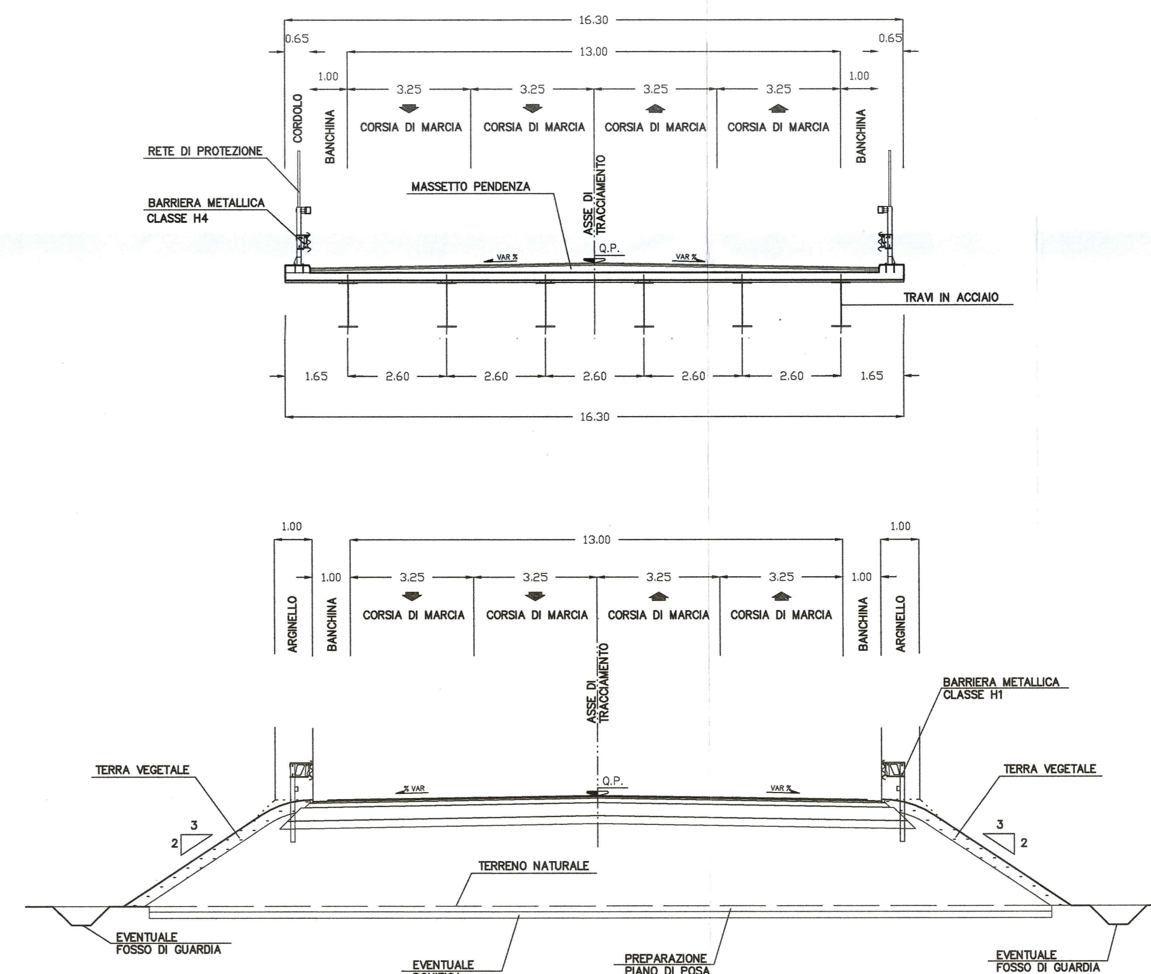
SEZIONE TIPO scala 1:100
