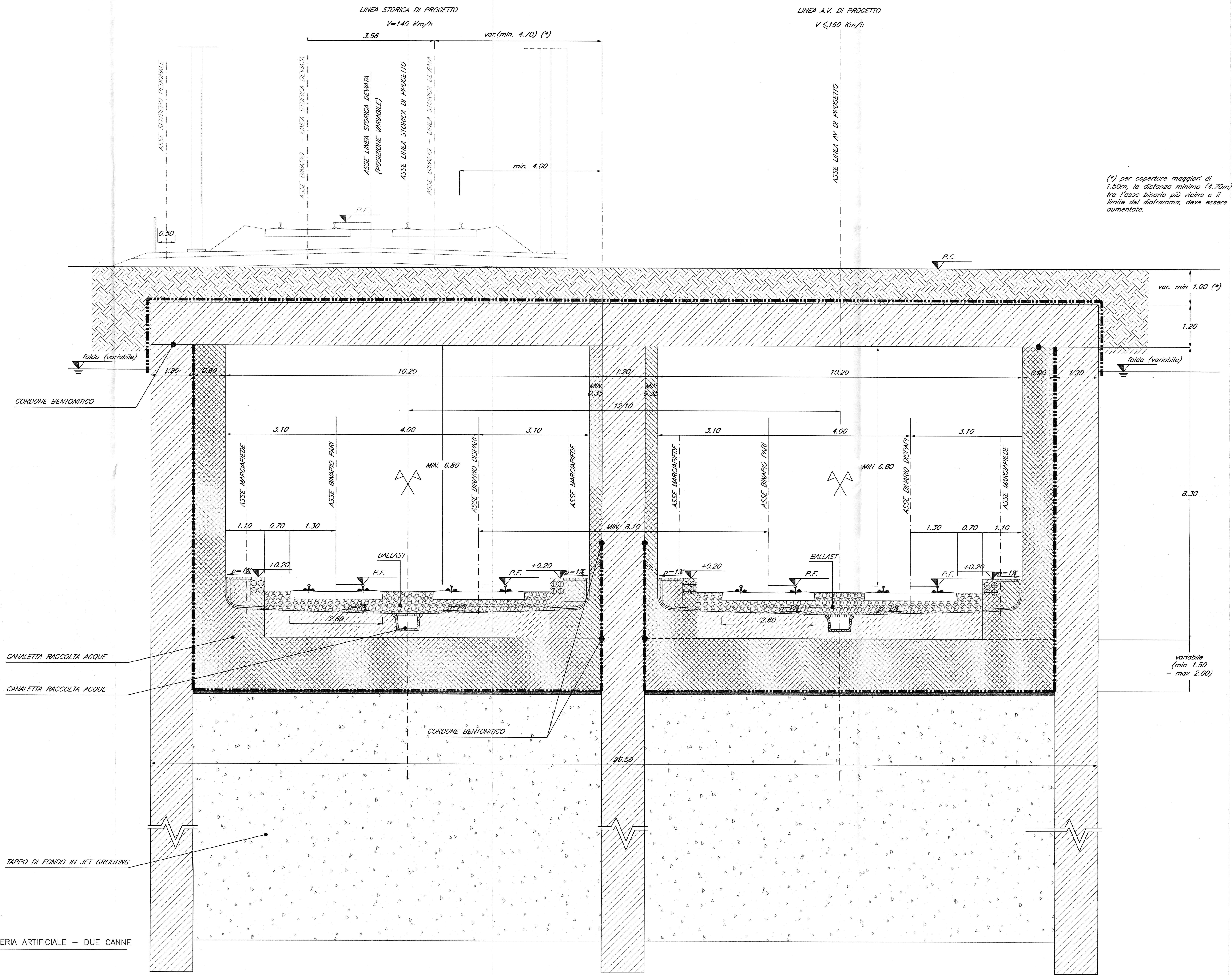
SEZIONE TIPO IN AFFIANCAMENTO IN GALLERIA ARTIFICIALE - DUE CANNE SCATOLARE scala 1:50
