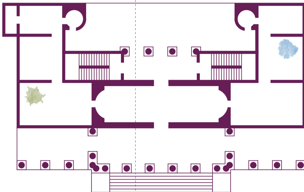
Palazzo Chiericati PIANO TERRA
