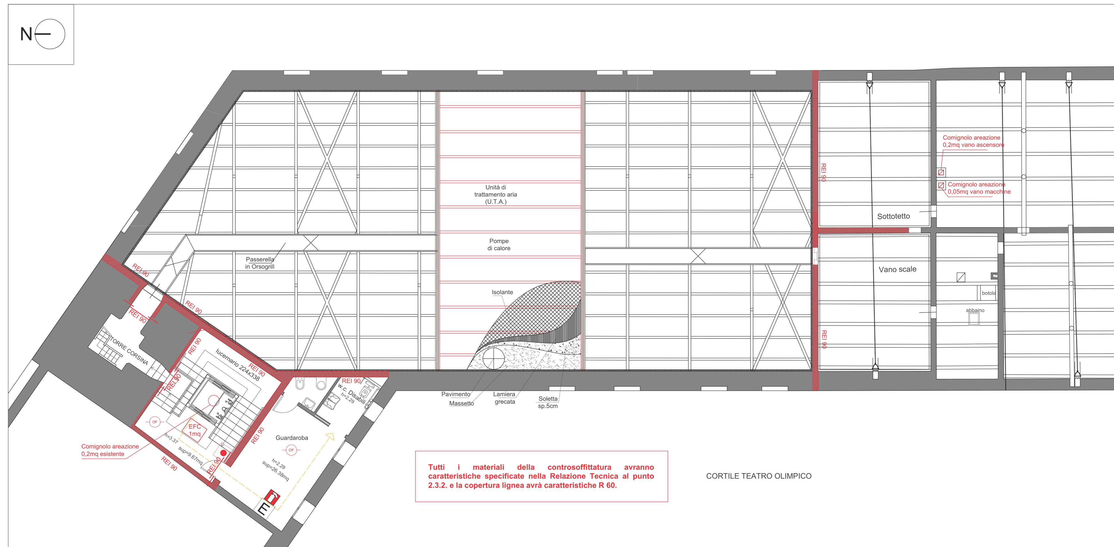
PIANTA PIANO SOTTOTETTO _ Scala 1:100
